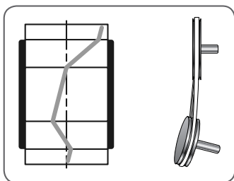
Рис 8 Отображение комбинации трех видов несоосности
