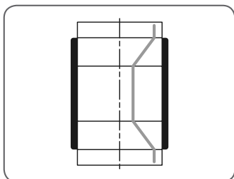
Fig 11 Remskivor med horisontellt vinkelfel och parallellförskjutning samtidigt
