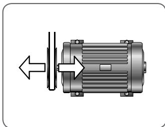
Fig 14 Parallell uppriktning
