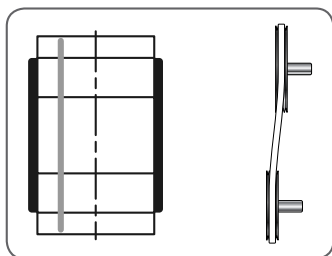
Рис 7 Отображение параллельной несоосности
