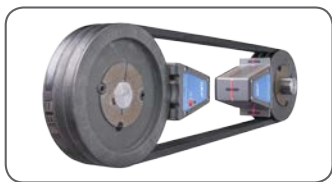
图4 激光单元装到皮带轮槽的示意图
