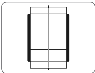
Fig 15 Perfekt uppriktade remskivor
