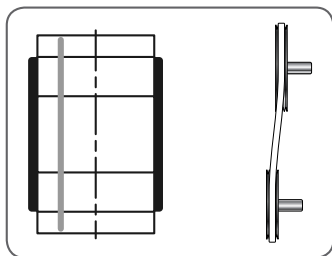
Fig 7 Weergave van de parallelle uitlijnfout
